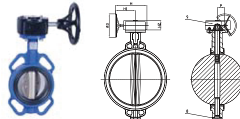
(DBV1603WG), PN16
